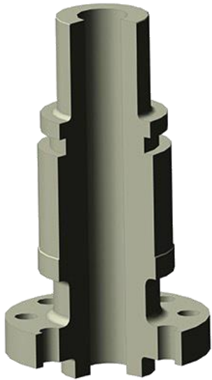
ИМЗ-14.275.10 Вал вертлюга барабана ГТ установки МК-20Т
